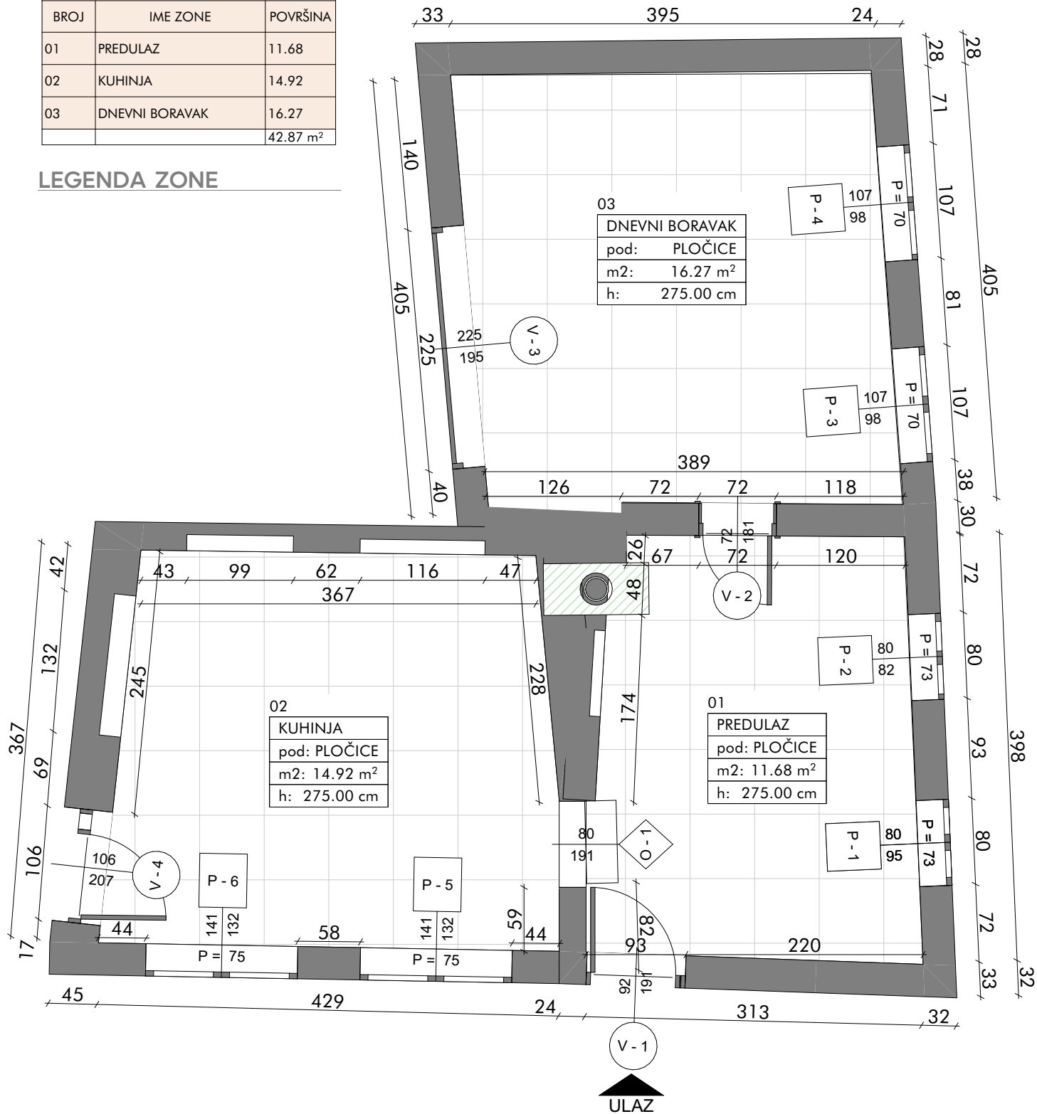
0. Tlocrt – postojeće stanje
