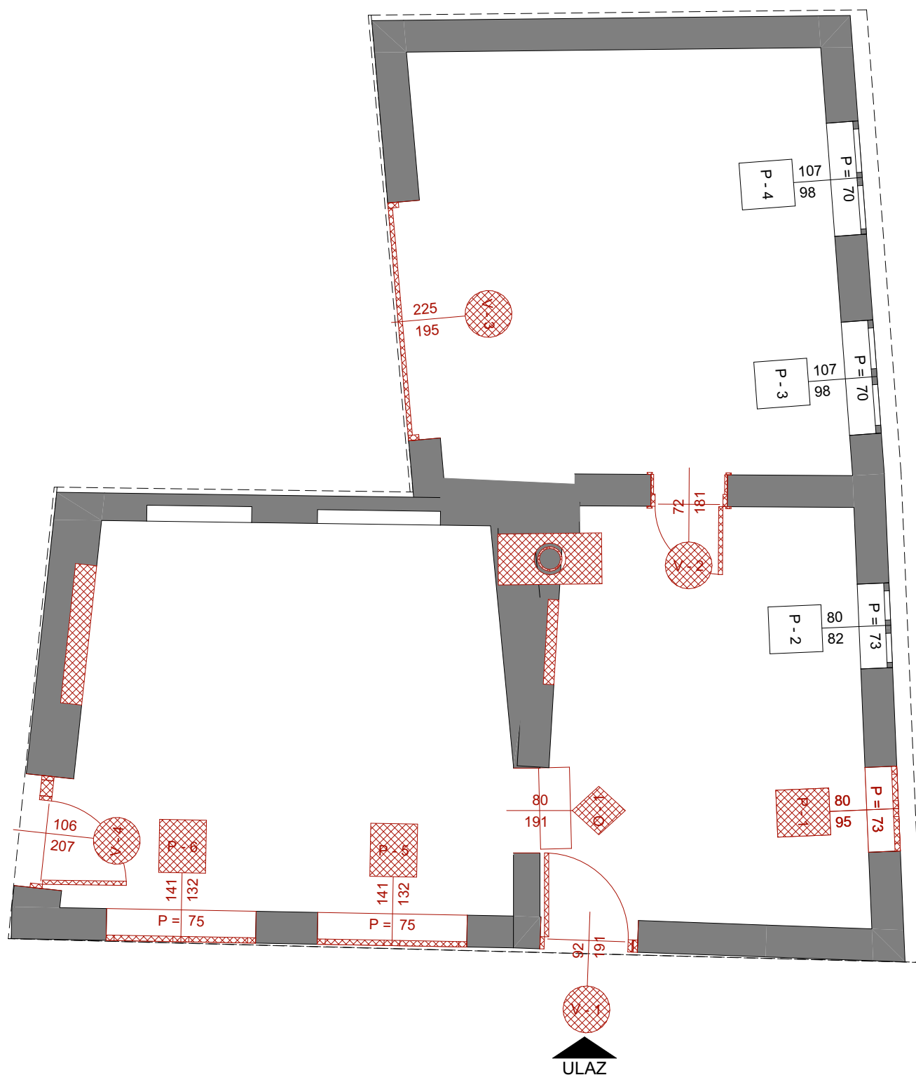
0. Tlocrt – rušenje
