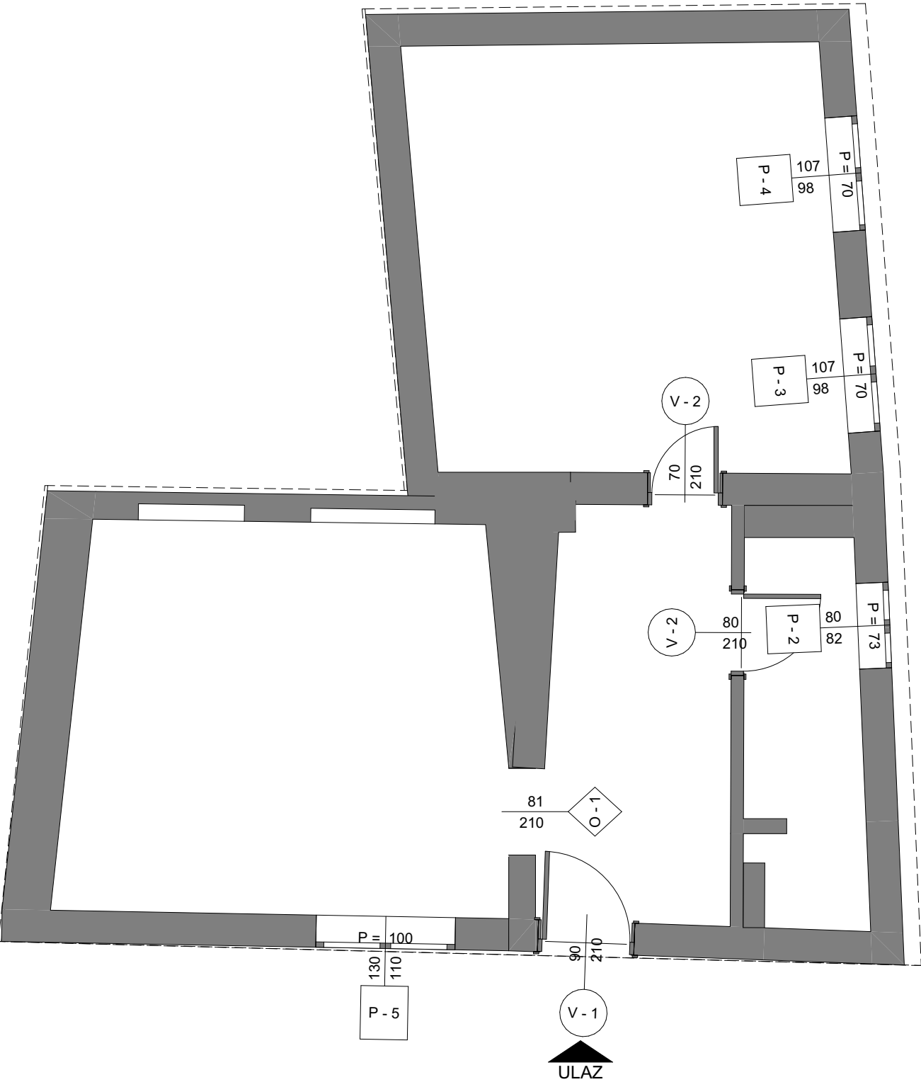
0. Tlocrt - planirano stanje 1:50
