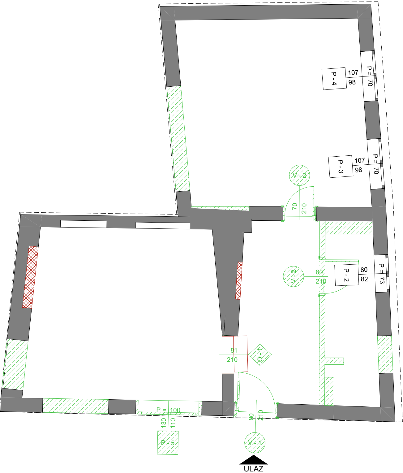
0. Tlocrt - promjena 1:50
