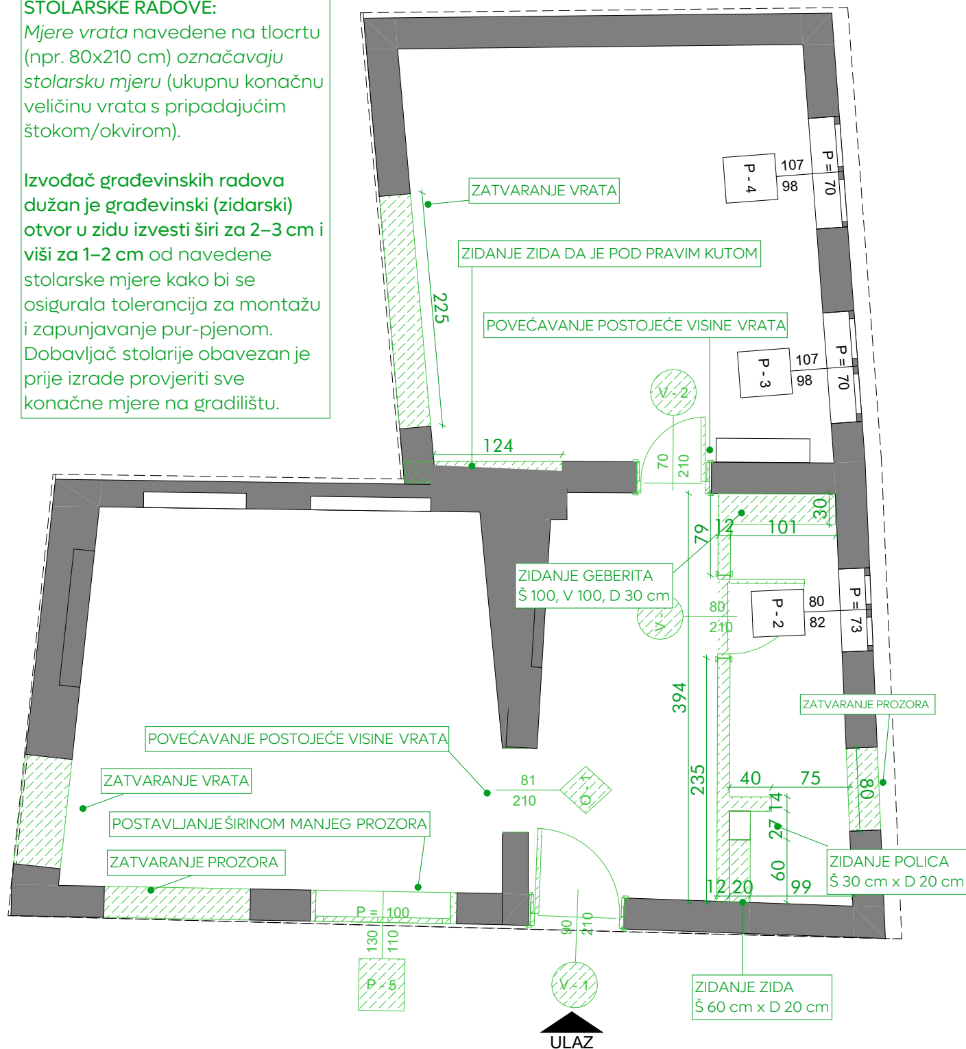
0. Tlocrt – zidanje
